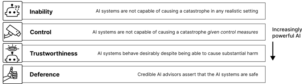
FIG. 3.2 Les briques de base à partir desquels construire une démonstration de la sécurité d'un composant ou sous-système intégrant de l'IA, classés par niveau de capacité de l'IA. Un argumentaire basé sur l'incapacité conçoit les IA comme ne disposant pas des moyens leur permettant de provoquer une catastrophe (notons que le terme accident n'est pas utilisé, car il présuppose la non-malveillance de l'IA). Un argumentaire basé sur la notion de contrôle démontre que différents dispositifs de détection et de contrôle empêchent l'IA de provoquer une catastrophe. Un argumentaire basé sur la confiance justifiée suppose que le concepteur ou intégrateur système peut démontrer que l'IA assurera toujours la fonction de sécurité voulue, même en l'absence de mécanismes qui permettraient de contrôler sa capacité à provoquer une catastrophe. Un argumentaire basé sur la déférence à l'autorité s'appuie sur l'assurance fournie par une IA-conseil jugée crédible que le composant à base d'IA ne provoquera pas une catastrophe. Source : [Clymer et al. 2024].
